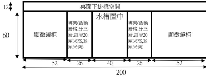
學生實驗桌下面平面圖(水槽置中)
